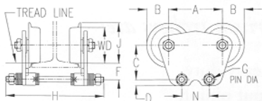
Push Type Trolley 1/4, 1/2 & 1 Ton
